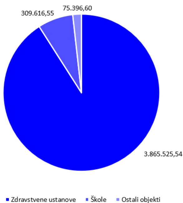
Grafikon 4. Prikaz potrošnje ekstra lakog lož ulja po skupinama objekata
