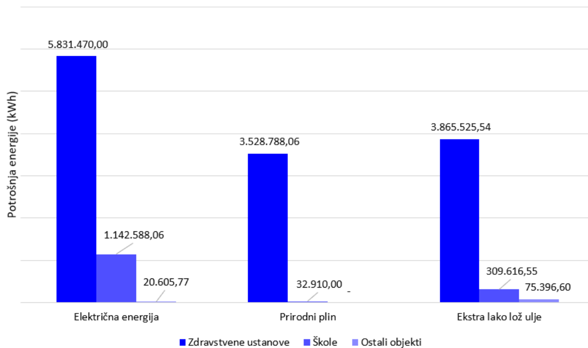
Grafikon 1. Prikaz ukupne potrošnje energije po skupinama objekata
